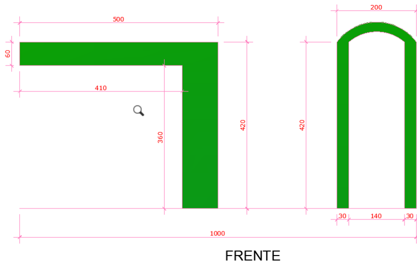
Imagem 05: Dimensões da frente do Stand.
