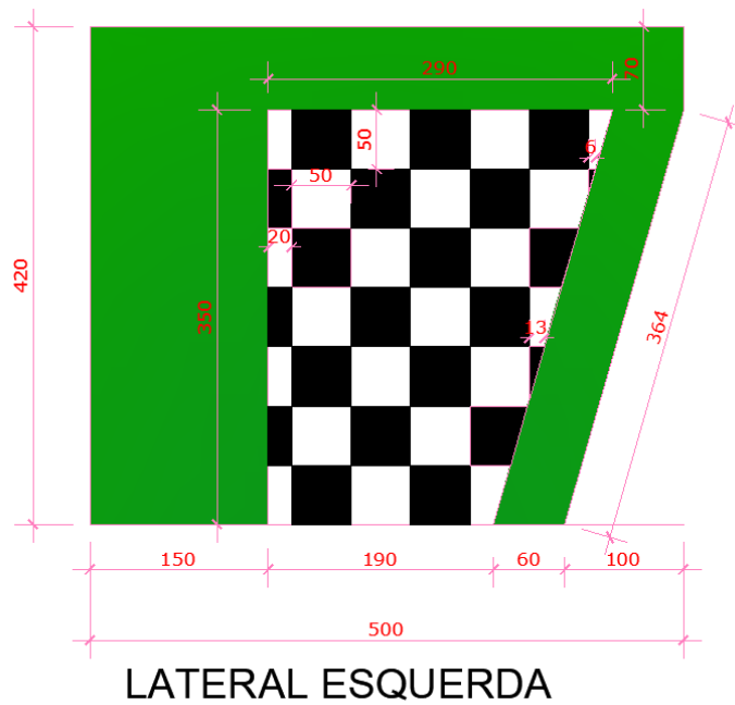
Imagem 06: Dimensões da lateral esquerda, com elementos vazados.
